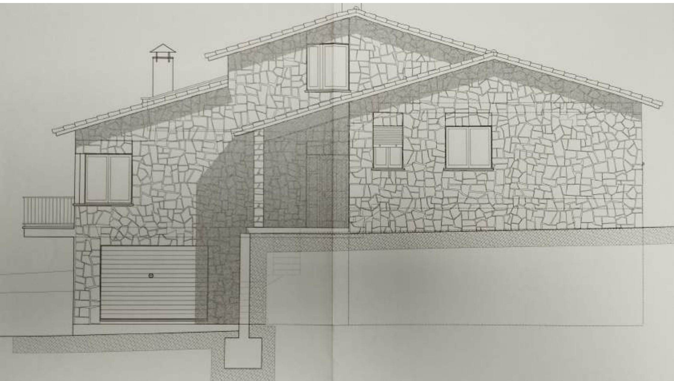
FAÇANA NORD
